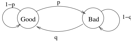
Fig. 2. Error model
